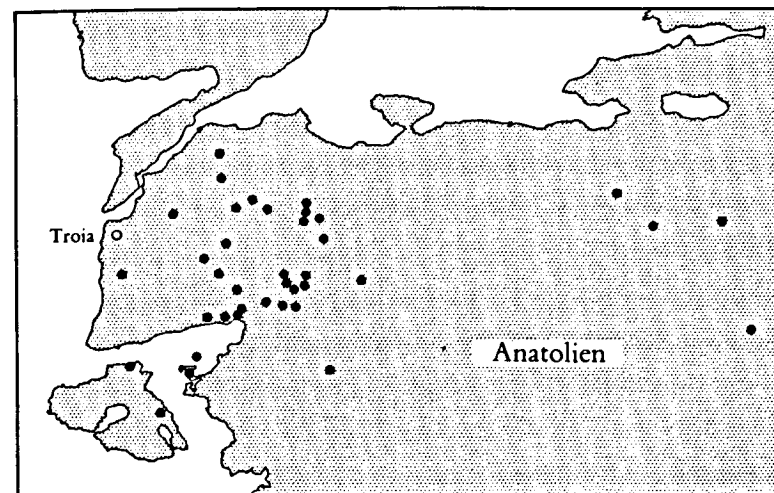
Die Verteilung von Erzlagern im Nordwesten Anatoliens zeigt, daß die Troas besonders reich an metallischen Bodenschätzen ist (nach Wagner u. a. 1985).
