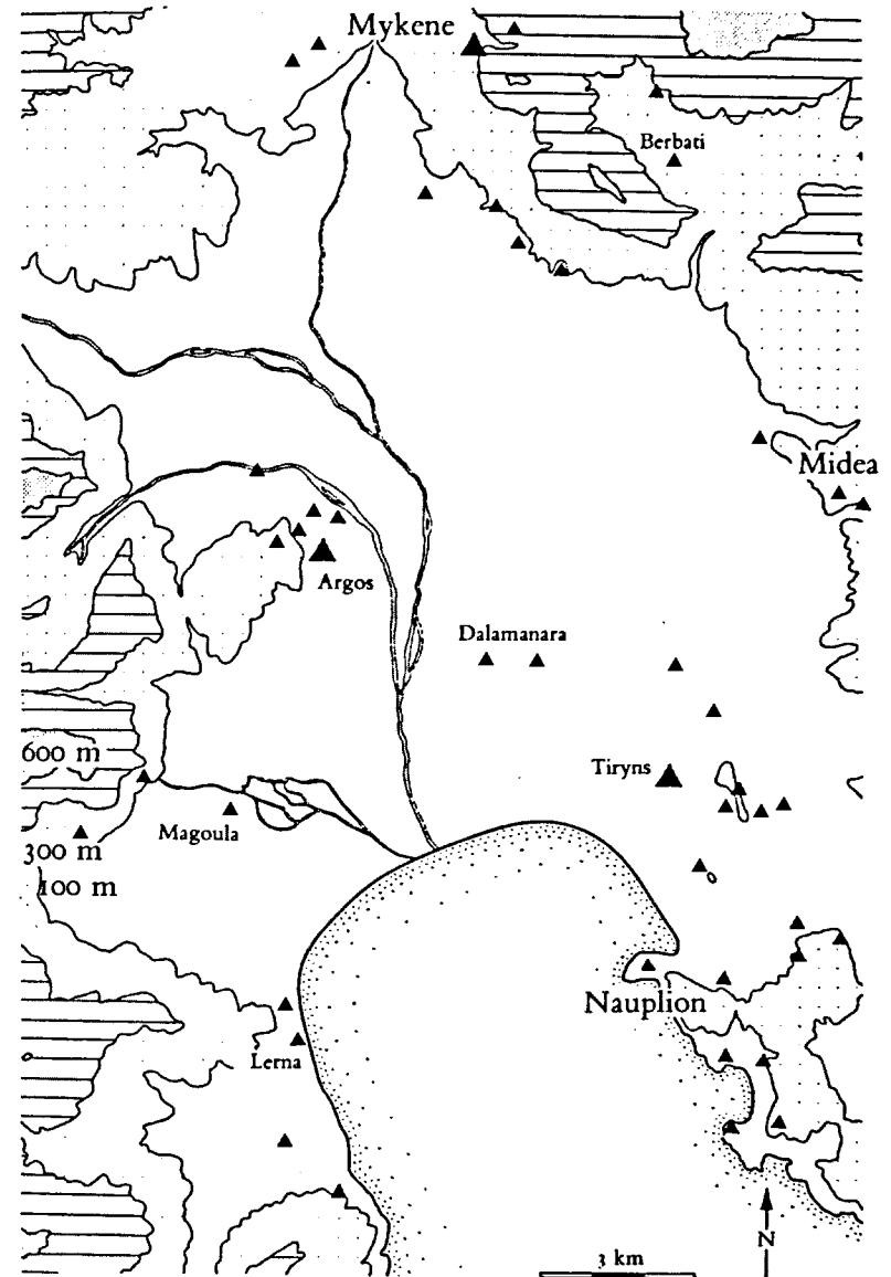
Siedlungen der Spätbronzezeit in der argivischen Ebene (nach Kilian 1982).
