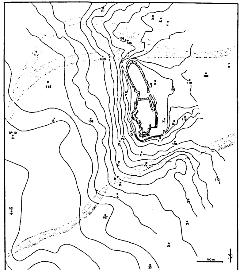
Karte des Gebiets um die Burg von Tiryns. Sie zeigt, an welchen Stellen während der geoarchäologischen Untersuchung Kernbohrungen (Punkte und Dreiecke) sowie Ausgrabungen (Quadrate) durchgeführt wurden. (Nach Zangger 1991a)
