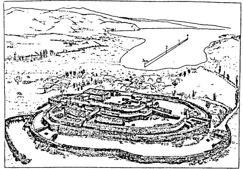
Die neolithische Siedlung Dimini wurde auf einem Hügel direkt an der Küste errichtet. Im Laufe der Zeit füllte sich die flache Bucht vor der Ansiedlung mit Ablagerungen. Es ist denkbar, daß die Ablagerungen auf Abholzung und die daraus resultierende Bodenerosion zurückgingen. Heute verläuft die Küste drei Kilometer weiter meerwärts (aus Zangger 1991b).
